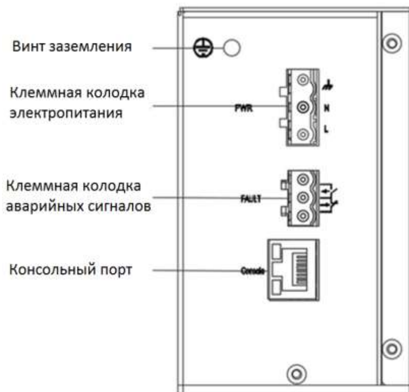
Рис. 3. Верхняя панель SEWM-RB-3GC-HI-XX
