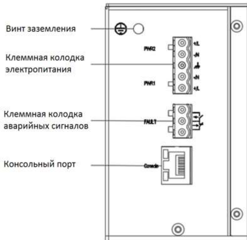
Рис. 2. Верхняя панель SEWM-RB-3GC-24E-24E
