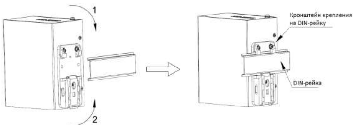
Рис. 8. Монтаж на DIN-рейку №2
