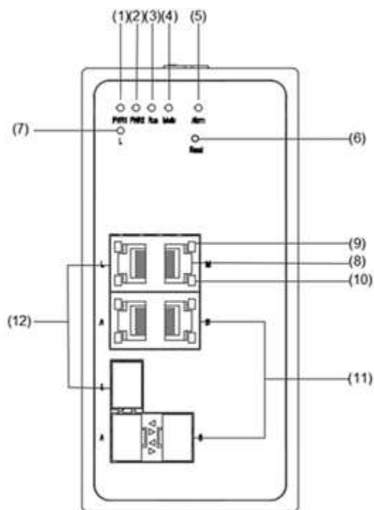
Рис. 1. Передняя панель
