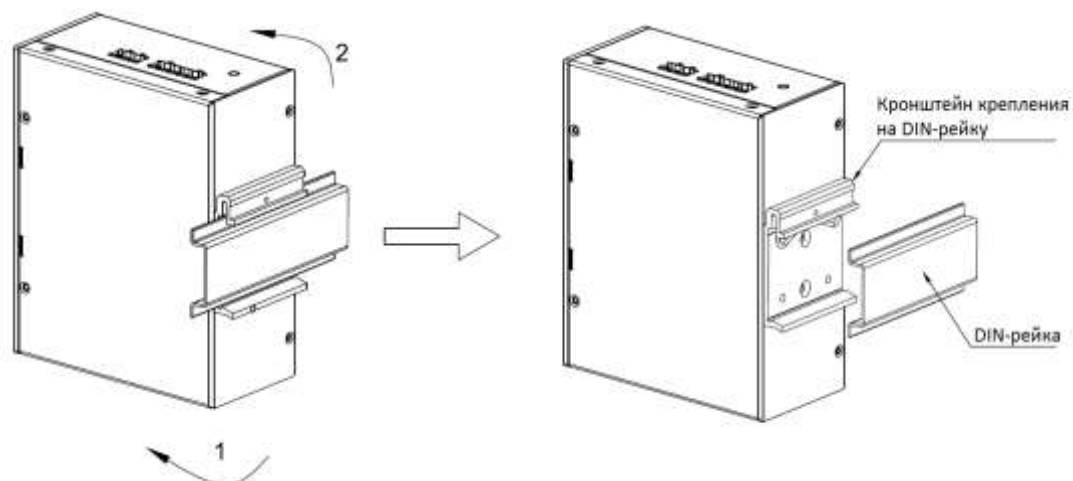
Рис. 7. Демонтаж с DIN-рейки, вариант №1
