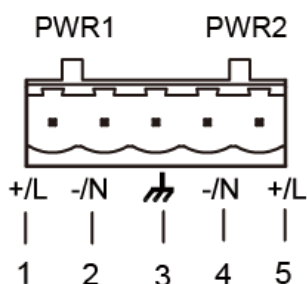
Рис. 19. 5-ти пиновая клеммная колодка питания 5,08 мм
