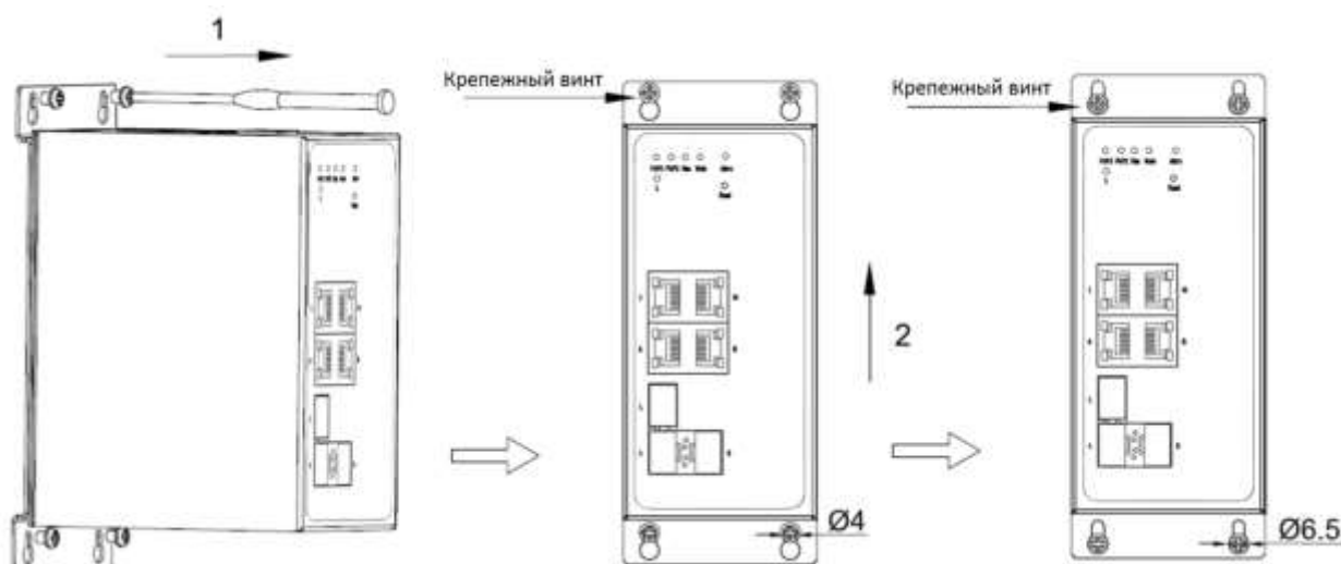
Рис. 10. Демонтаж с плоской поверхности
