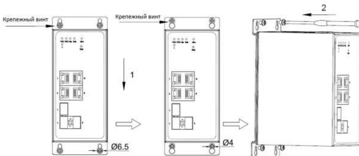
Рис. 9. Монтаж на плоскую поверхность
