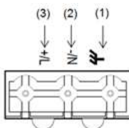
Рис. 20. 3-х пиновая клеммная колодка питания 7,62 мм
