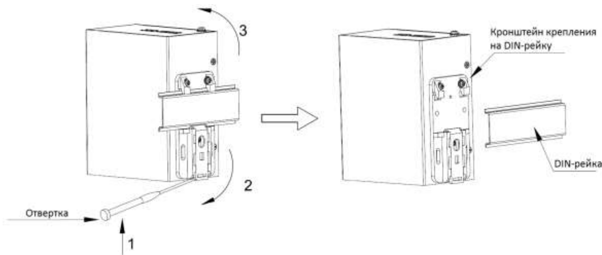
Рис. 9. Демонтаж с DIN-рейки, вариант №2
