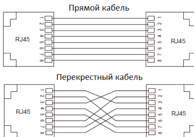
Рис. 13. Схема кабелей
