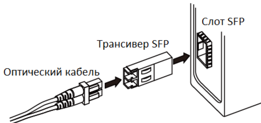
Рис.16. Подключение трансивера SFP
