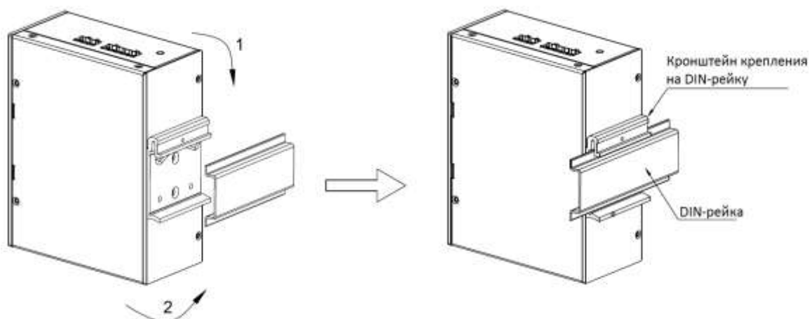
Рис. 6. Монтаж на DIN-рейку, вариант №1
